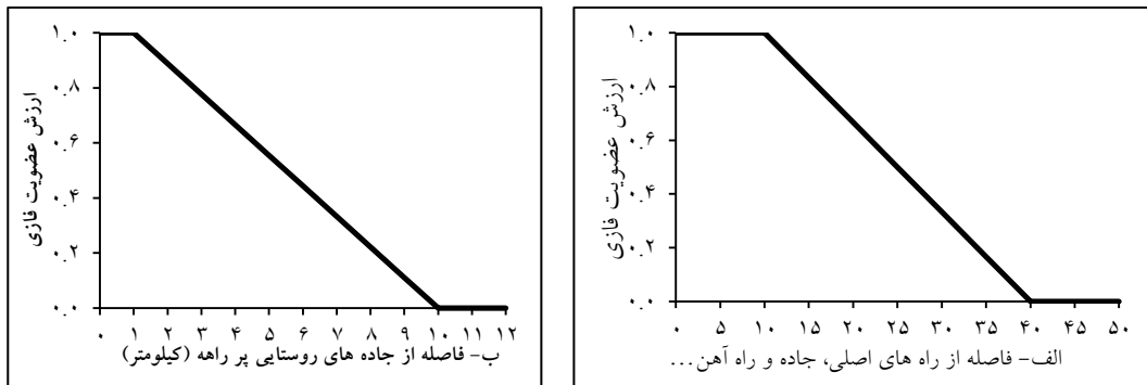
نمودار ۳. توابع عضویت فازی دسترسی به جاده و خطوط ارتباطی جهت احداث مزارع خورشیدی
