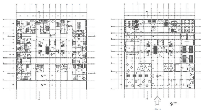
شکل ۸. (سمت راست) پلان اقامتگاه بین راهی طبقه همکف، (سمت چپ) پلان اقامتگاه بین راهی طبقه اول مأخذ: نگارندگان
