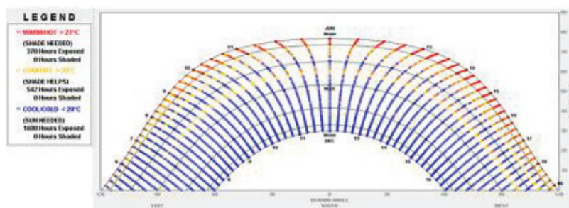
شکل ۴(الف). محدوده شرایط گرم، سرد و آسایش در حد فاصل ساعات طلوع تا غروب خورشید
