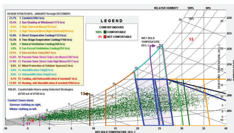
شکل ۶. توصیه های طراحی بر اساس نیازهای حرارتی بروندی و آسایش در نمودار
