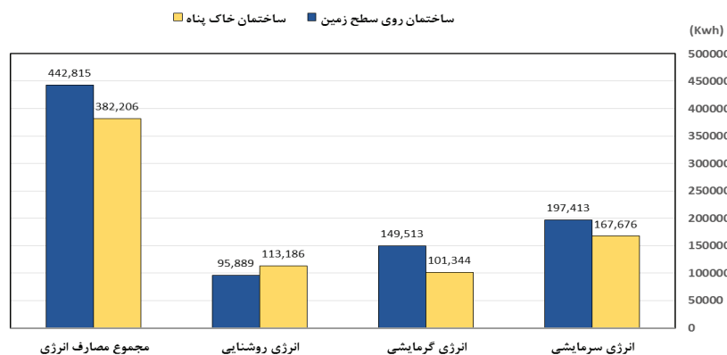
شکل ۱۰. مقایسه مصرف انرژی سالانه در اقامتگاه بین راهی مدل خاک پناه و روی سطح زمین
