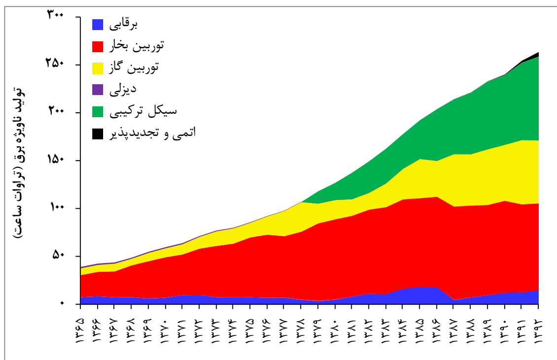
نمودار (۱): تولید ناویژه برق به تفکیک نیروگاه‌های مختلف در ایران (آمار تفصیلی ۹۲، توانیر ۹۳)
