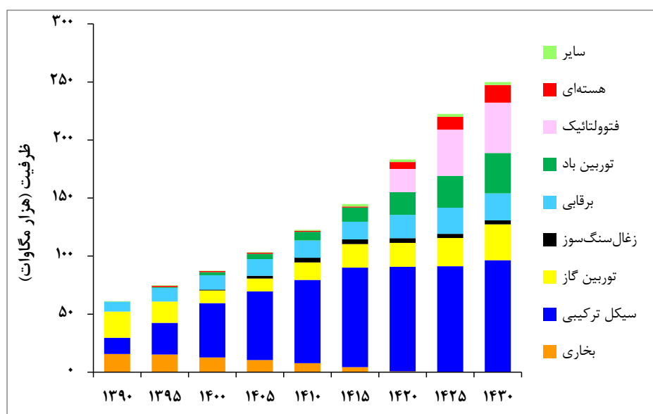
نمودار (۲): روند بهینه کل ظرفیت نصب شده نیروگاهی در سناریوی مرجع (سایر: مجموع نیروگاه‌های دیزلی، توربین انبساطی، پیل سوختی، زمین گرمایی، حرارتی-خورشیدی و زیست توده)
