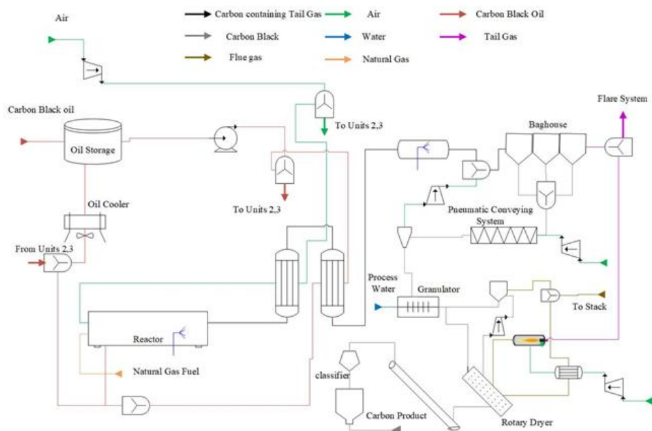
شکل ۲. فرآیند تولید دوده صنعتی دوده فام (۴، ۵)
