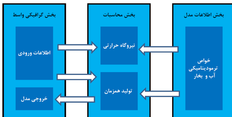
شکل ۲. فلودیاگرام ساختار نرم افزار DE-TOP
