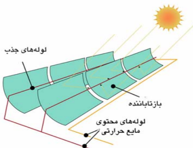
شکل (۷) : شمای کلی از عملکرد نیروگاه خورشیدی سهموی خطی
