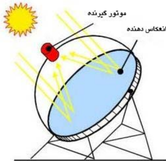
شکل (۹): شمای کلی از عملکرد دیش استرلینگ (گزارش CSP، آژانس بین‌المللی انرژی، ۲۰۱۲)
