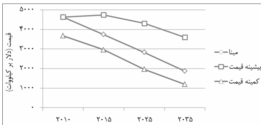
شکل (۳): پیش‌بینی هزینه سرمایه‌گذاری فناوری CSP
