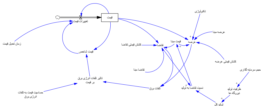
شکل ۲ نمودار جریان تحلیل تلفات انرژی برق
