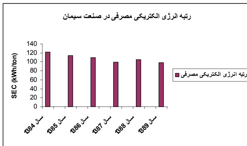
نمودار ۲. میزان مصرف انرژی الکتریکی ویژه در کارخانه سیمان در طی ۶ سال
