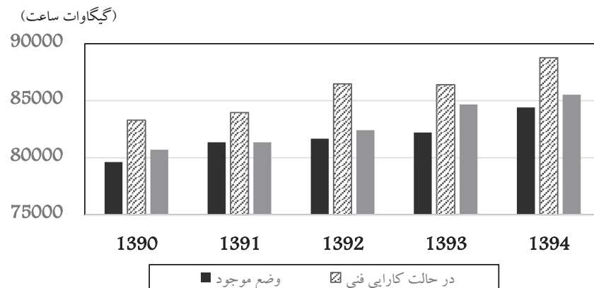
نمودار ۱. مقایسه روند تولید نیروگاه‌های حرارتی منتخب (۱۳۹۰-۱۳۹۴)
