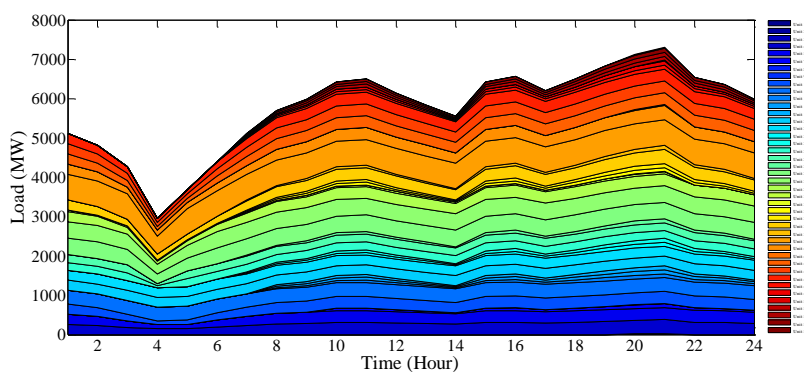
شکل ۸. نحوه توزیع توان بین واحدهای حرارتی در سیستم ۱۱۸ باس ۵۴ واحد IEEE (سناریو ۴)
