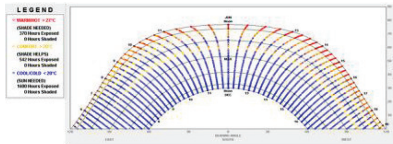
شکل ۴(الف). محدوده شرایط گرم، سرد و آسایش در حد فاصل ساعات طلوع تا غروب خورشید در شهرستان شاهرود (زمستان و بهار)
