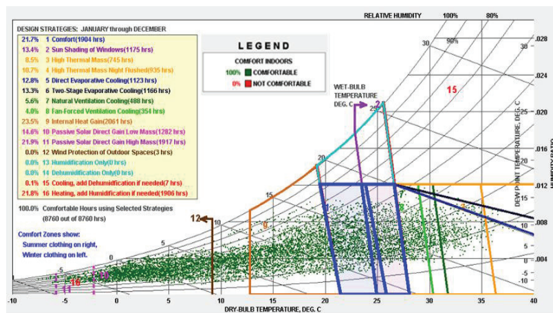
شکل ۶. توصیه های طراحی بر اساس نیازهای حرارتی برومتری و آسایش در نمودار
