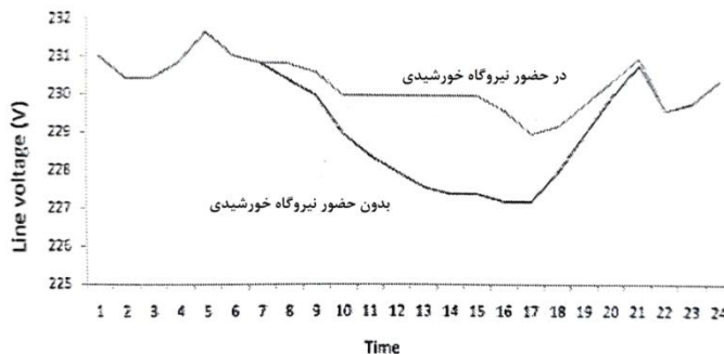
شکل ۶: نمودار پروفیل ولتاژ شبکه در نقطه اتصال نیروگاه خورشیدی
