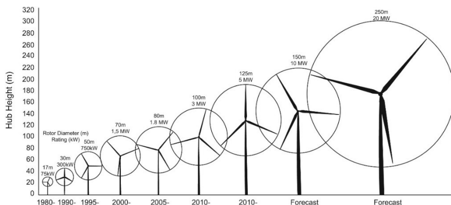
شکل ۳: اندازه‌های مختلف پره‌ها و پایه توربین‌های بادی (Abbasi et al., ۲۰۱۴)
