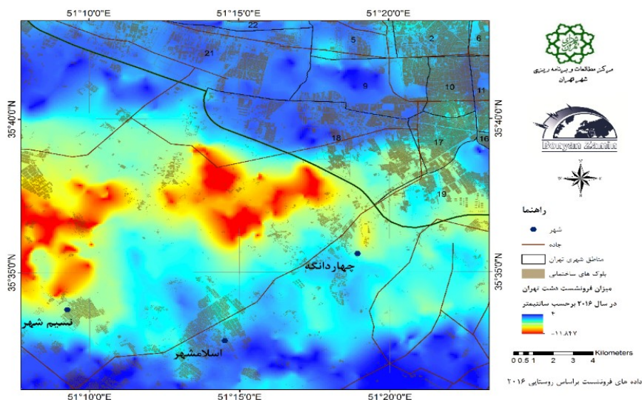
شکل ۶: نقشه فرونشست زمین در تهران، مرکز مطالعات شهر تهران منبع: مرکز مطالعات و برنامه ریزی شهر تهران، ۱۳۹۸
