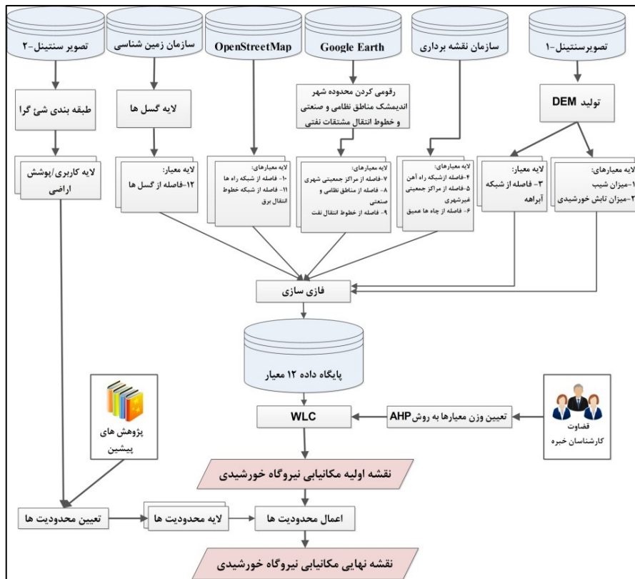
شکل ۲. فلوجارت مواد و روش پژوهش
