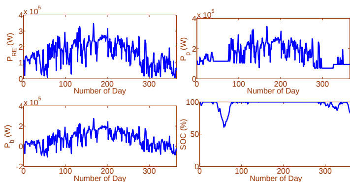
نمودار ۹. منحنی توان تولید شده منابع تجدیدپذیر بادی و خورشیدی P_{RE} ، توان تولید شده سیستم ترکیبی P_p ، ورودی / خروجی سیستم بانک باتری P_b و تغییرات SOC برای ساختمان C
