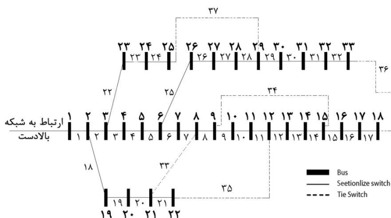
شکل ۴ شبکه مورد مطالعه ۳۳ شینه
