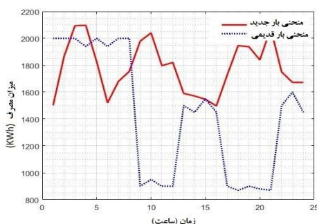
شکل ۱۳. منحنی مقایسه‌ای مصرف روزانه کارخانه سیمان
