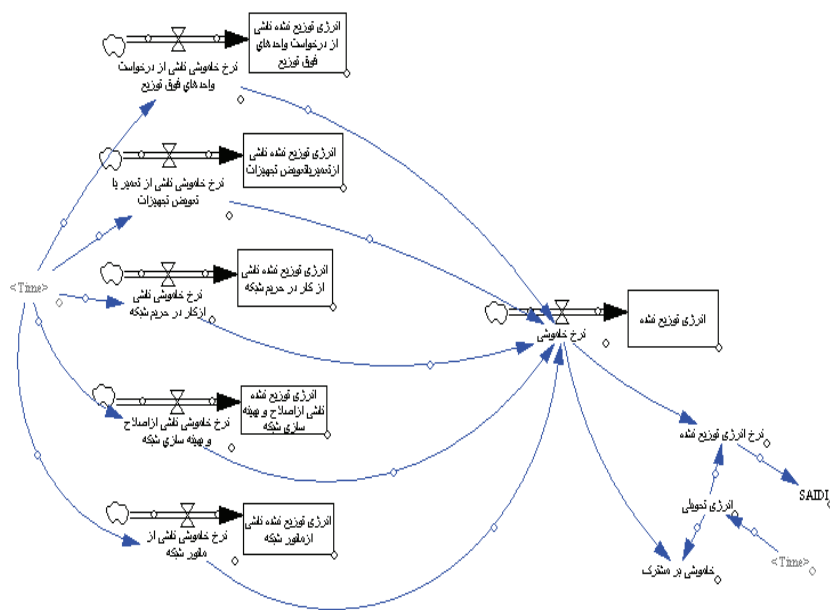
شکل ۴. نمودار انباشت جریان خاموشی با برنامه (ارزوی توزیع نشده)
