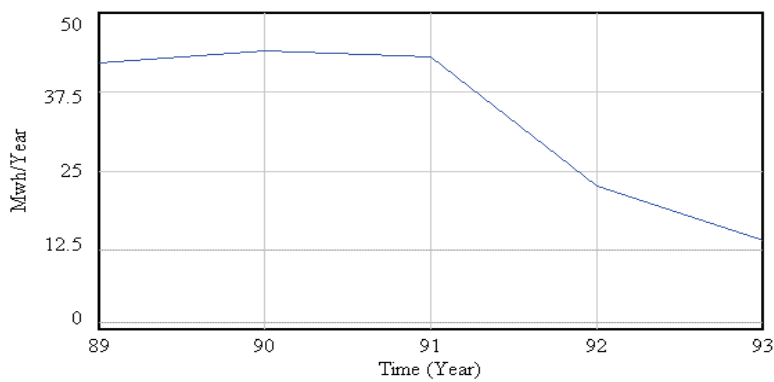
شکل ۵. ارزوی توزیع نشده ناشی از شرایط نامساعد جوی (مگاوات ساعت)
