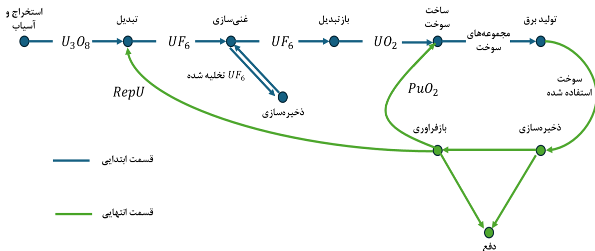
شکل (۱): چرخه سوخت هسته‌ای ۲۲
