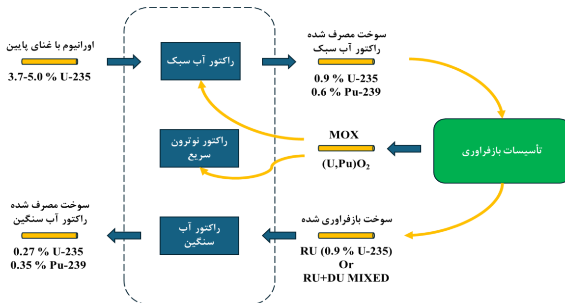
شکل (۳): برنامه‌ریزی چین در چرخه سوخت هسته‌ای ۴۵
